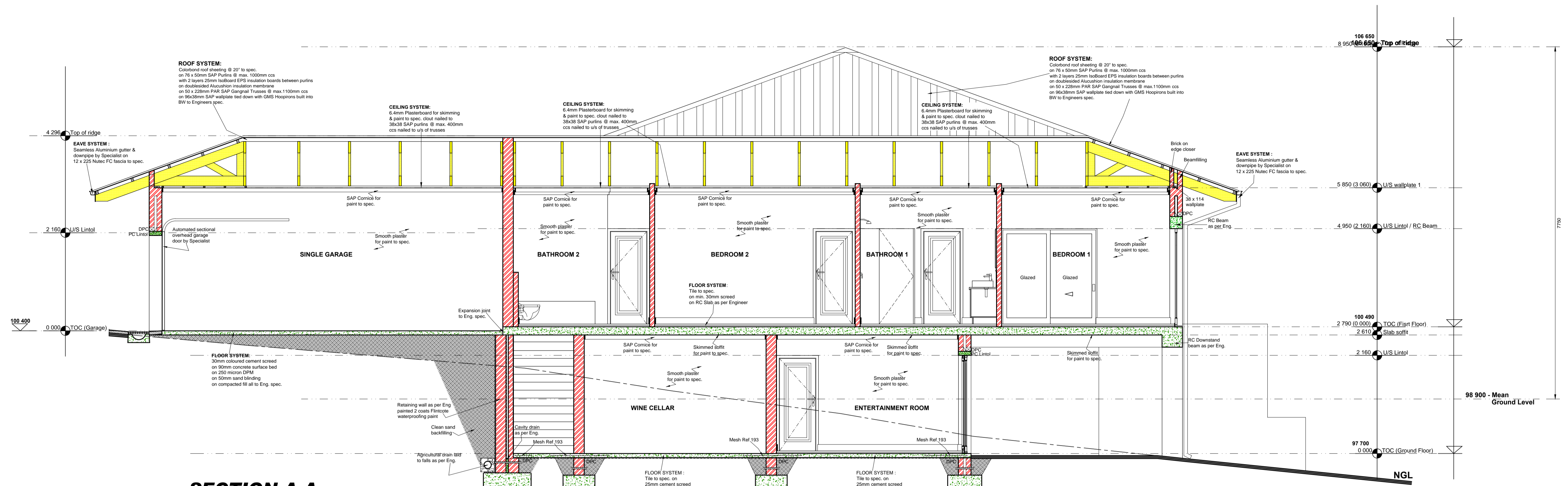
SECTION A-A
